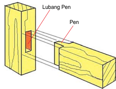
Gambar 10. Sambungan pen dan lubang
