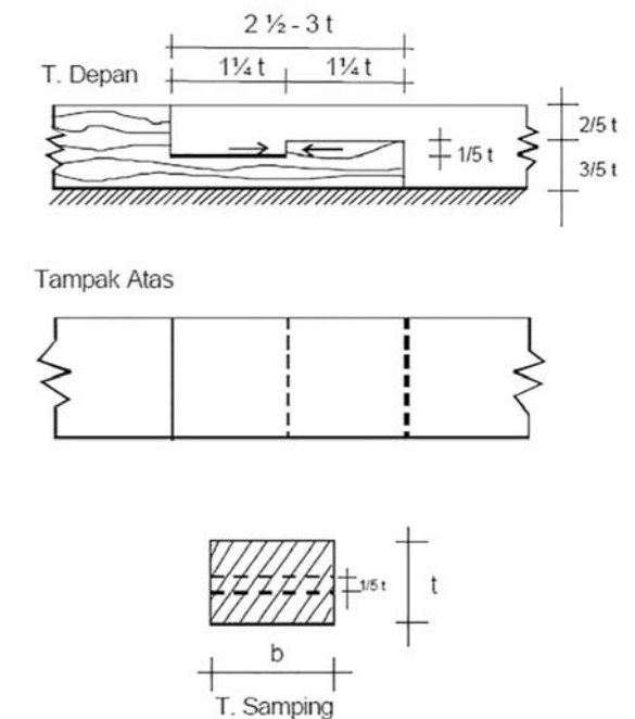
Gambar 15. Sambungan bibir lurus
