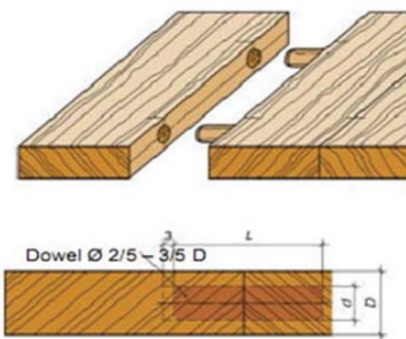
Gambar 12. Sambungan dowel kayu
