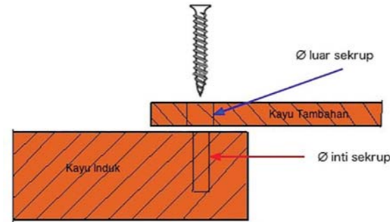
Gambar 17. Sambungan dengan sekrup
