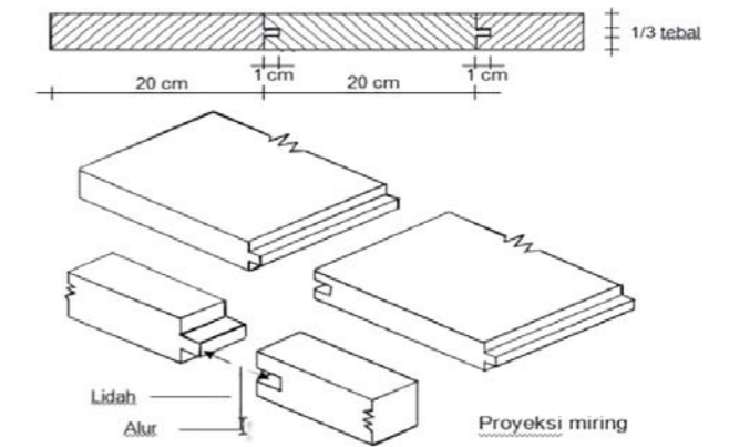
Gambar 14. Sambungan melebar alur dan lidah
