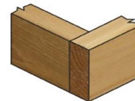
Gambar 7. Sambungan biasa
