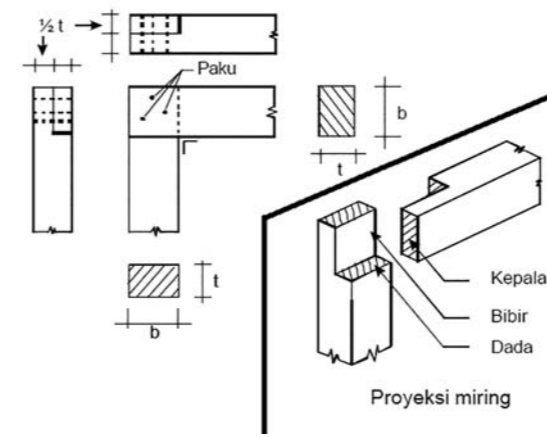
Gambar 13. Sambungan takikan lurus
